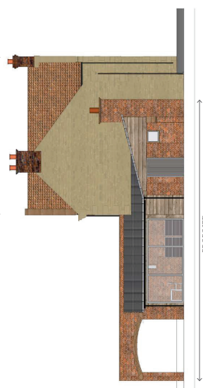
Elevation DD 1:100@A1
